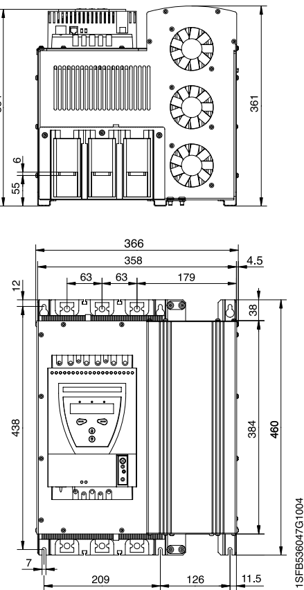
PSTB370 ... 470
