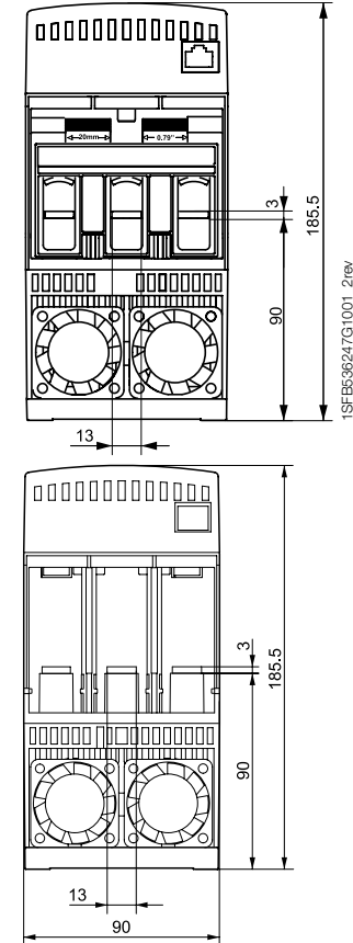
PSE18 ... 105
