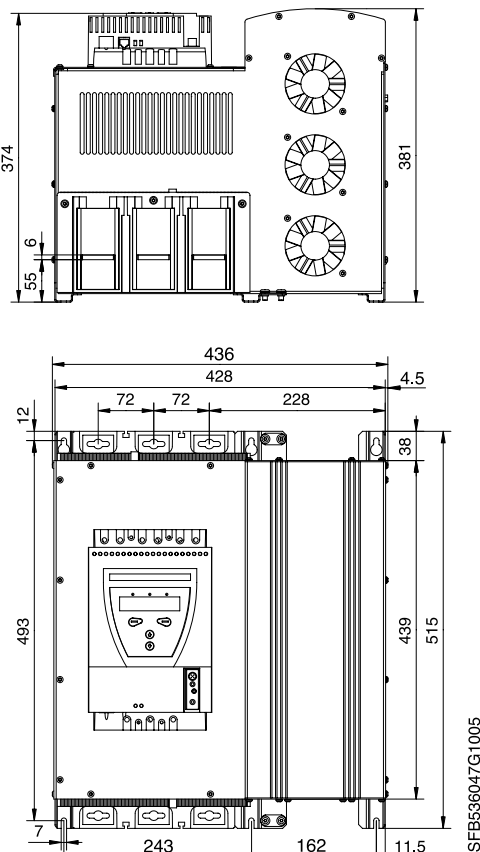
PSTB570 ... 1050
