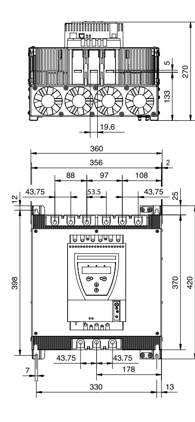
PST175 ... 300
