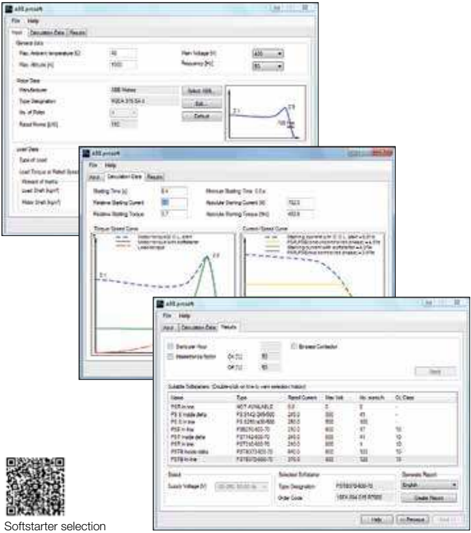
Softstarter selection
